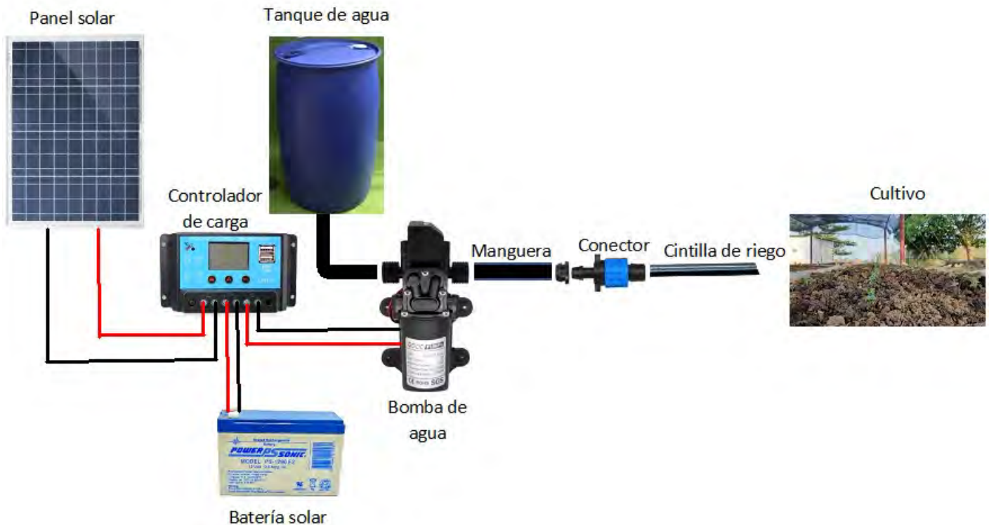
Figura 2. Representación gráfica del sistema de riego solar fotovoltaico. (Elaboración propia, 2021).
